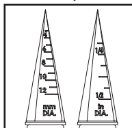
Mesures du diamètre d'alésoir de carrosserie conique
