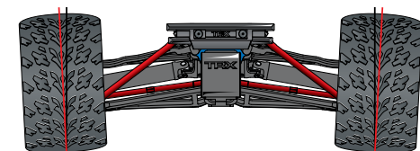
Inclinación positiva Las ruedas se inclinan hacia afuera, lejos del chasis
