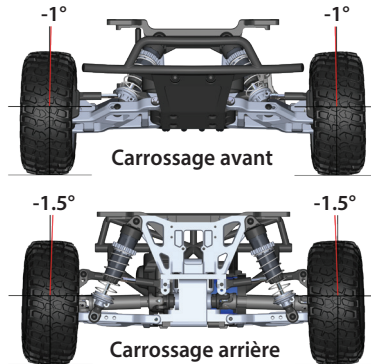
Carrossage arrière
