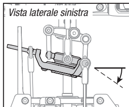
Elevatore alzato
