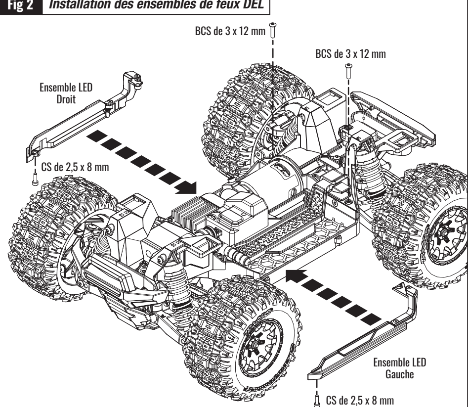
Fig 2 Installation des ensembles de feux DEL
