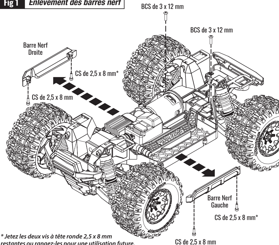
Fig 1 Enlèvement des barres nerf
