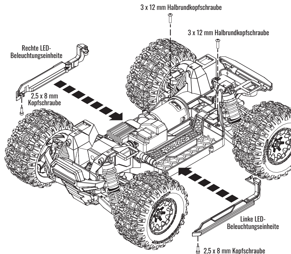
Fig 2 Installation der LED-Unterbodenbeleuchtungseinheiten
