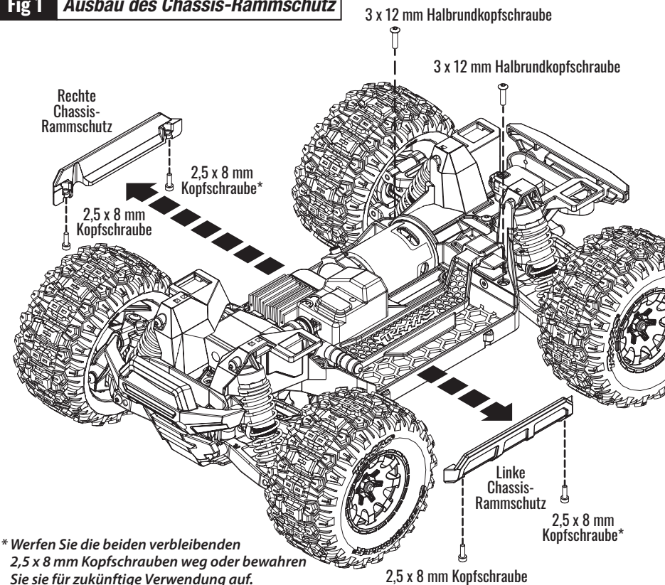
Fig 1 Ausbau des Chassis-Rammschutz
