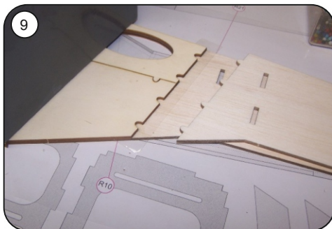
9 Das zweite Rumpfvorderteil deckungsgleich auf das erste legen und fixieren ( spätere Rumpfaussenseiten gegeneinander ) Rumpfseitenteil R3 ankleben, dabei auch auf Deckungsgleichheit am Rumpfende achten.
