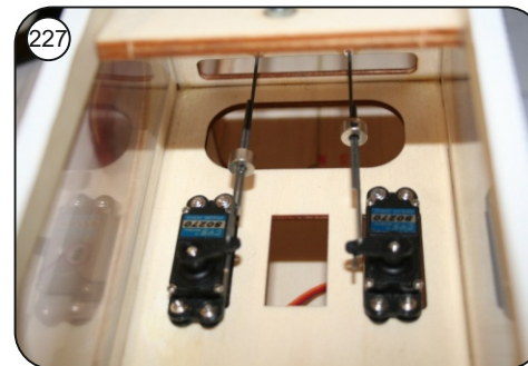
227 Z-Gestänge für die Servoanschlüsse herstellen, in die Servoarme einhängen und mit Stellringen mit den Ruderanlenkungen verbinden. Bowdenzugrohr im Spantendurchgang mit Epoxy sichern.
