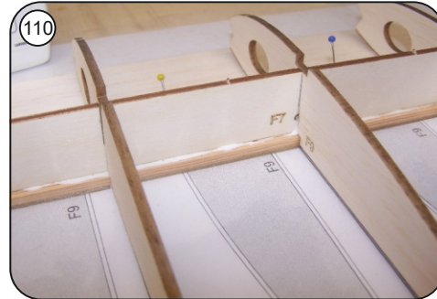
110 Holmgurt auf der gesamten Restlänge satt mit Holzleim einstreichen, Kammholzverlängerung an der Stossrippe einsetzen und die restlichen Rippen F9 einkleben.
