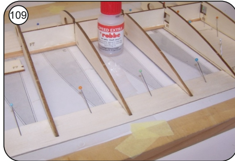
109 Rippe F8 und die ersten 3 Rippen F9 in den Kammholm F7, den Holmgurt und die unter Beplankung F4 einkleben.
