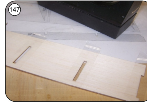
147 Steckungsslitze für die Rippensegmente von der Unterseite mit Tesafilm abkleben.
