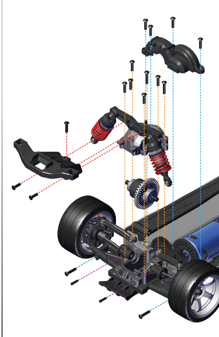
Retiro del diferencial trasero
