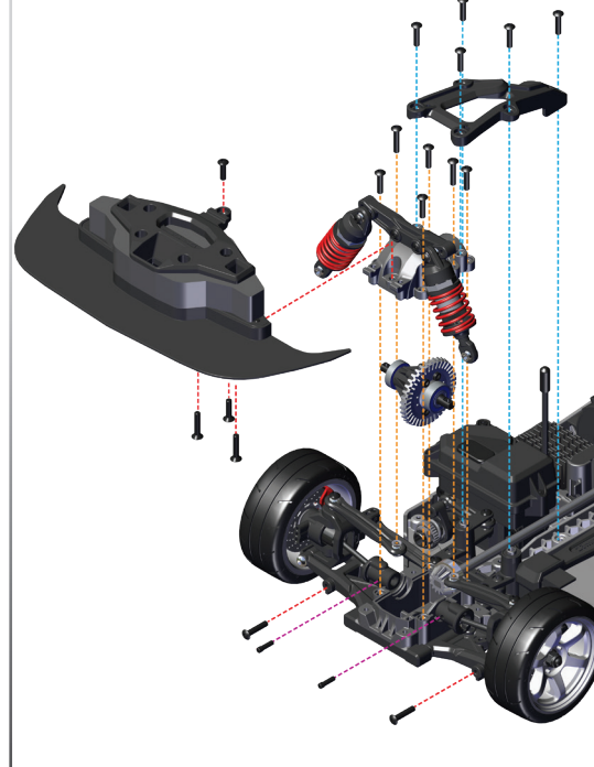
Retiro del diferencial delantero
