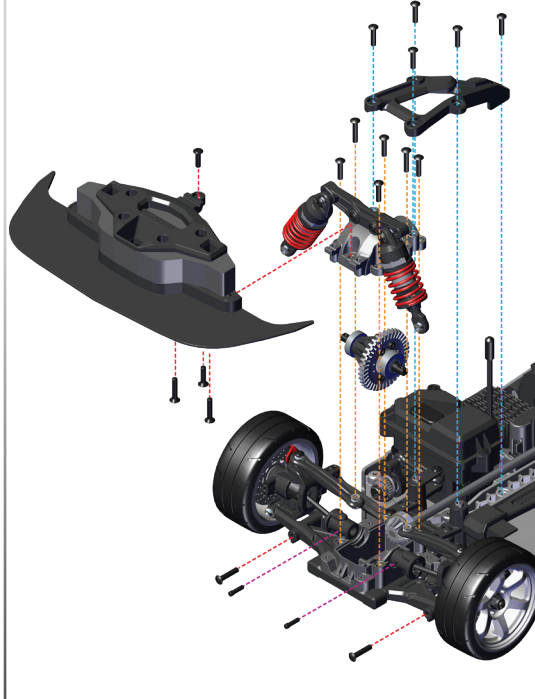
Démontage du différentiel avant
