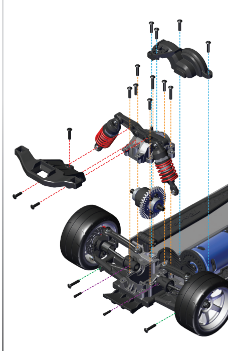
Démontage du différentiel arrière
