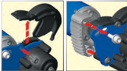
Ubicaciones de la estructura del motor
