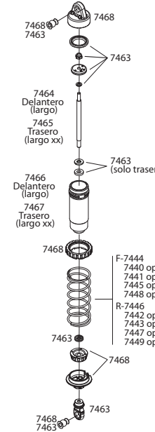
D. Instalación/extracción del pistón
