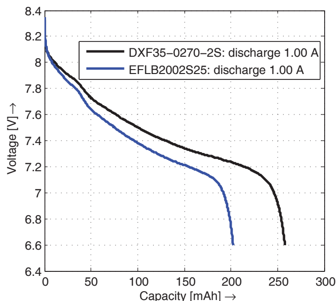
Obrázek: Typické vybíjecí charakteristika baterií E-Flite EFLB2002S25 a Duremax DXF35-0270-2S.
