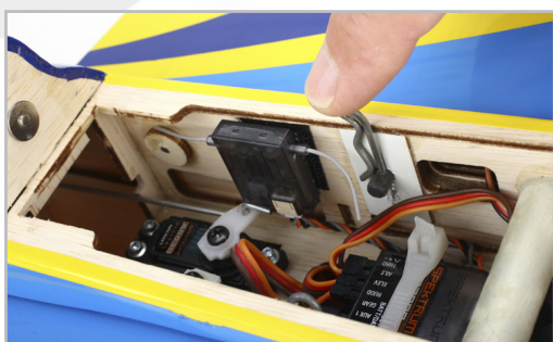
Dvoudílné křídlo je jištěno proti vysunutí pérovou pojistkou
