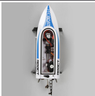
Elektronika i pohon jsou nainstalovány, motor s vodním chlazením, integrovaný přijímač/regulátor.
