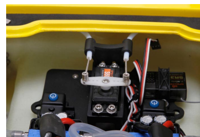
K řízení je použita RC souprava DX2E s přijímačem SR310 a voděodolným servem řízení SPMS605 9kg/cm s kovovými převody.
