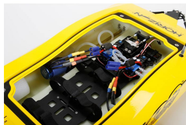
Vodou chlazené střídavé regulátory Dynamite 120A pro 2 - 6 článků LiPol baterií.
