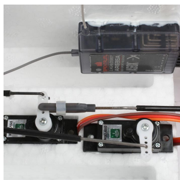
Nainstalovaný přijímač AR636A se stabilizací AS3X a funkcí SAFE s letovými módy Začátečnický, Pokročilý, a Zkušený
