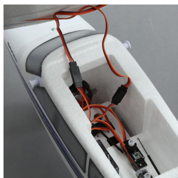
V trupu jsou nainstalována digitální serva pro ocasní plochy a příďovou nohu. pomocí kabelů se připojí serva křídélka.
