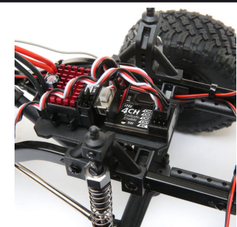
Nainstalován je přijímač ECX 2.4GHz a regulátor Dynamite® 60A WP FWD/REV.
