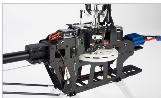
Kostra vrtulníku
