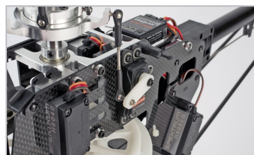
Rotorová hlava
