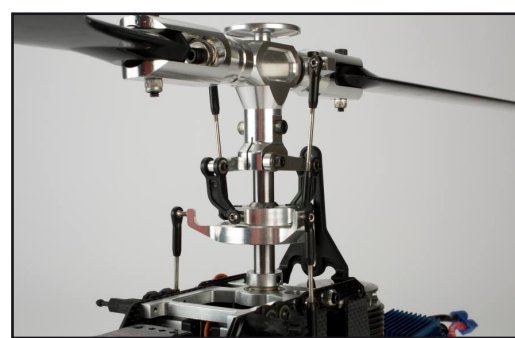
Rotorová hlava
