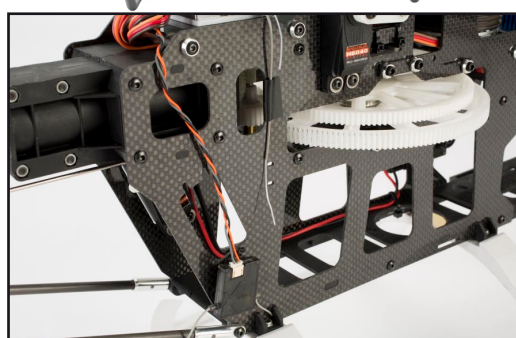
Kostra vrtulníku
