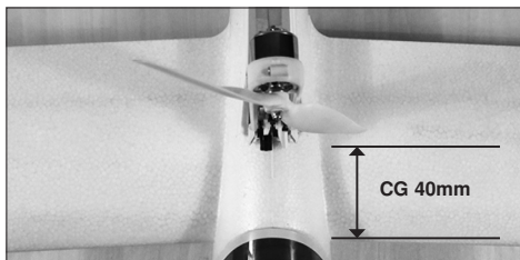
El centro de gravedad está a 40 mm. con el motor desplegado.
