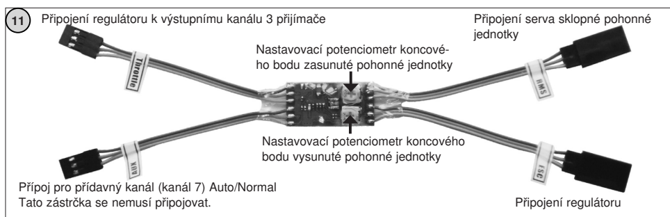
Obr. 11 – 1.1 Modul mixéru pro sklopnou pohonnou jednotku:
