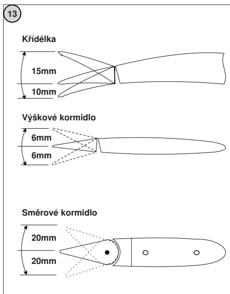
Obr. 13 Výchytky kormidel
