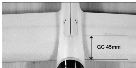
Poloha těžiště je 45 mm při zasunutí pohonné jednotce.
