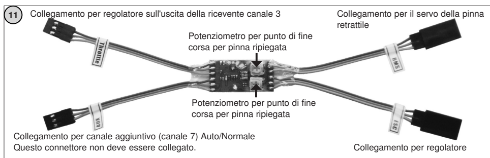
Figura 11 – 1.1 Modulo Mixer per la pinna retrattile:
