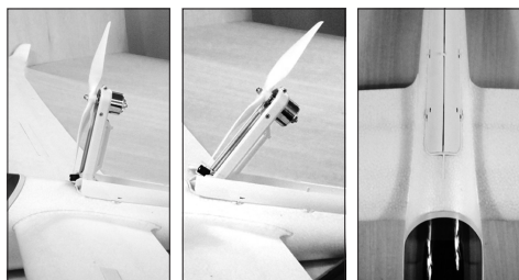
Figura 11 – 1.1 Modulo Mixer per la pinna retrattile:
