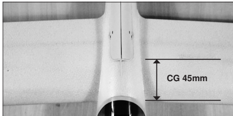
El centro de gravedad está a 45 mm. con el motor plegado.
