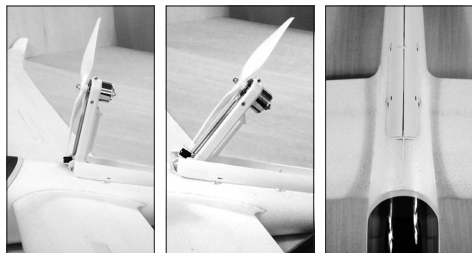
Fig. 11 – 1.1 Module de mixage de l'entraînement escamotable:
