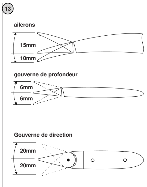
Fig. 13 Débattements des gouvernes
