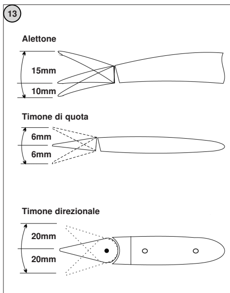
Figura 13 Escursione timoni
