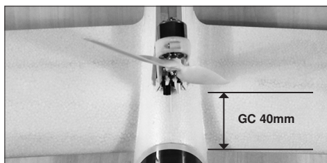
Poloha těžiště je 40 mm při vysunutí pohonné jednotce.
