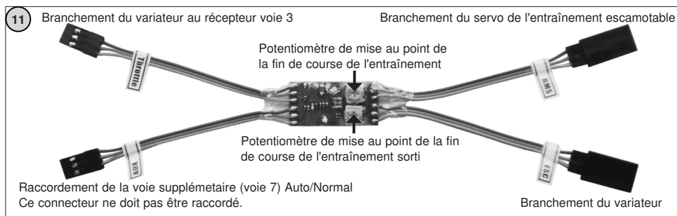
Fig. 11 – 1.1 Module de mixage de l'entraînement escamotable:
