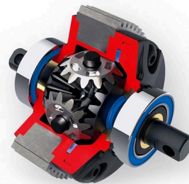
Diferenciál s kovovými převody
