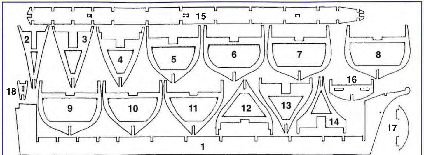
Tavola compensato - Plywood board - Sperrholzplatte - Planche contreplaqué - Plaat triplex - Tabla chapa
