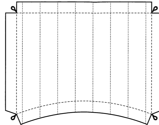
ALBERO DI MAESTRA MAIN MAST
