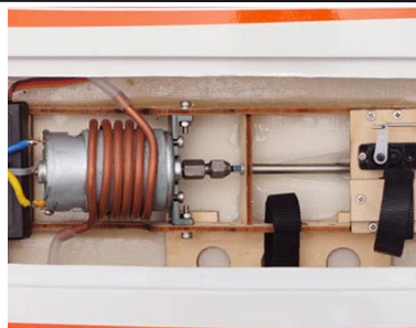
Nainstalovaný motor 550 s vodním chlazením, přijímač, vodou chlazený regulátor a servo řízení.
