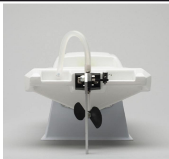
Rychlostní člun s charakteristickým profilem trupu Deep-V.
