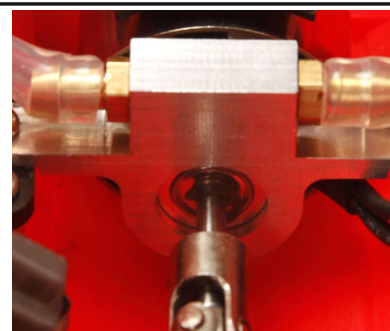
Střídavý 2950Kv vodou chlazený motor s oběžným pláštěm má na bloku motoru nainstalováno vodní chlazení.
