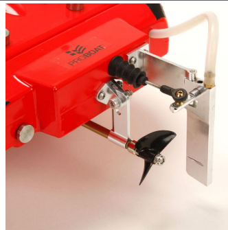
Lod' má nainstalováno Off-set kormidlo pro vynikající stabilitu a jízdní vlastnosti
