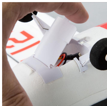
Pohonná LiPol baterie 280mAh 2S 30C se vkládá pod odklápěcí kryt na spodní části trupu.
