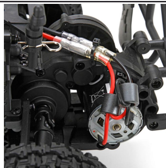
Motor Dynamite 15T je nainstalován za zadní nápravou, důraz je kladen na vyšší trakci.
