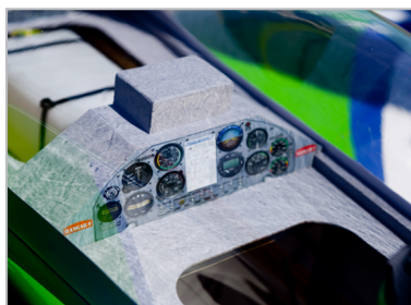
Detail kokpitu.
